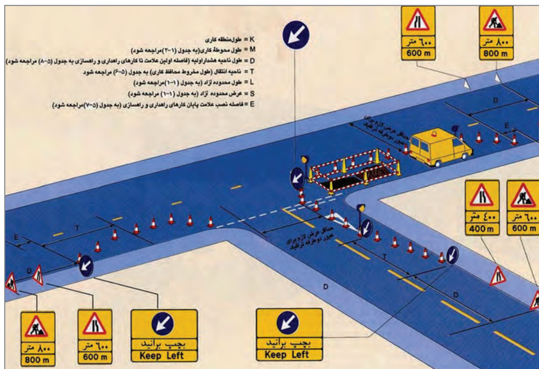
شکل ۳۰ - طرح علائم گذاری در تقاطع ها
