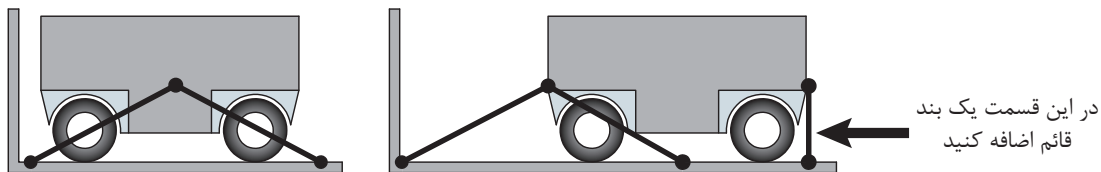
شکل ۲۰- روش بستن بند اضافی
