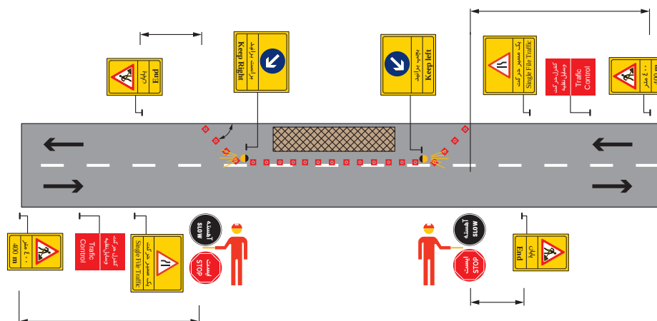
شکل ۲۳- طرح علامت گذاری برای کنترل ترافیک به وسیله علائم گردان (آهسته/ ایست) در یک راه دو خطه که یک خط آن بسته است.
